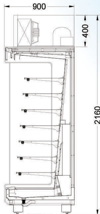
側視圖
