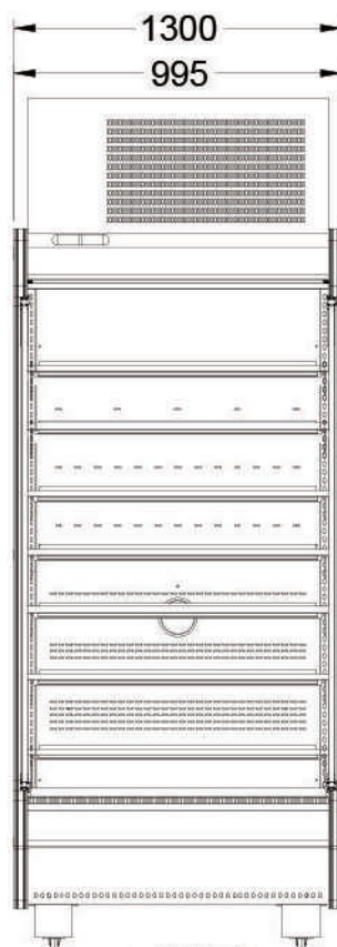
正視圖
